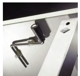
Cliphalterung: Die Kurbel wird einsatzbereit in der praktischen Clip-Halterung unter dem Tisch verstaut.
