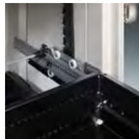
High-Tec im Büro: Vollauszüge mit Parallelsteuerung, End-Selbst-Einzug und Auszugssperre. Auf Wunsch auch mit Soft-Einzugsdämpfern.
