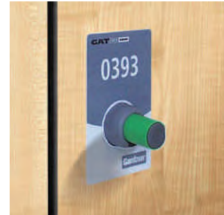
GAT 6000 B-Schloss: Elektronisches Schließsystem mit Druckfunktion und verschiedenen Formen der Datenträger-Integration.
